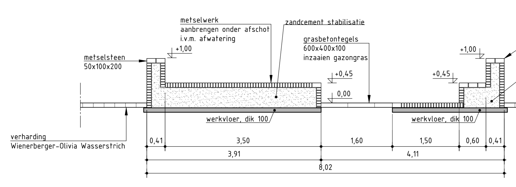
DWARSPROFIEL A-A SCHAAAL 1:50
