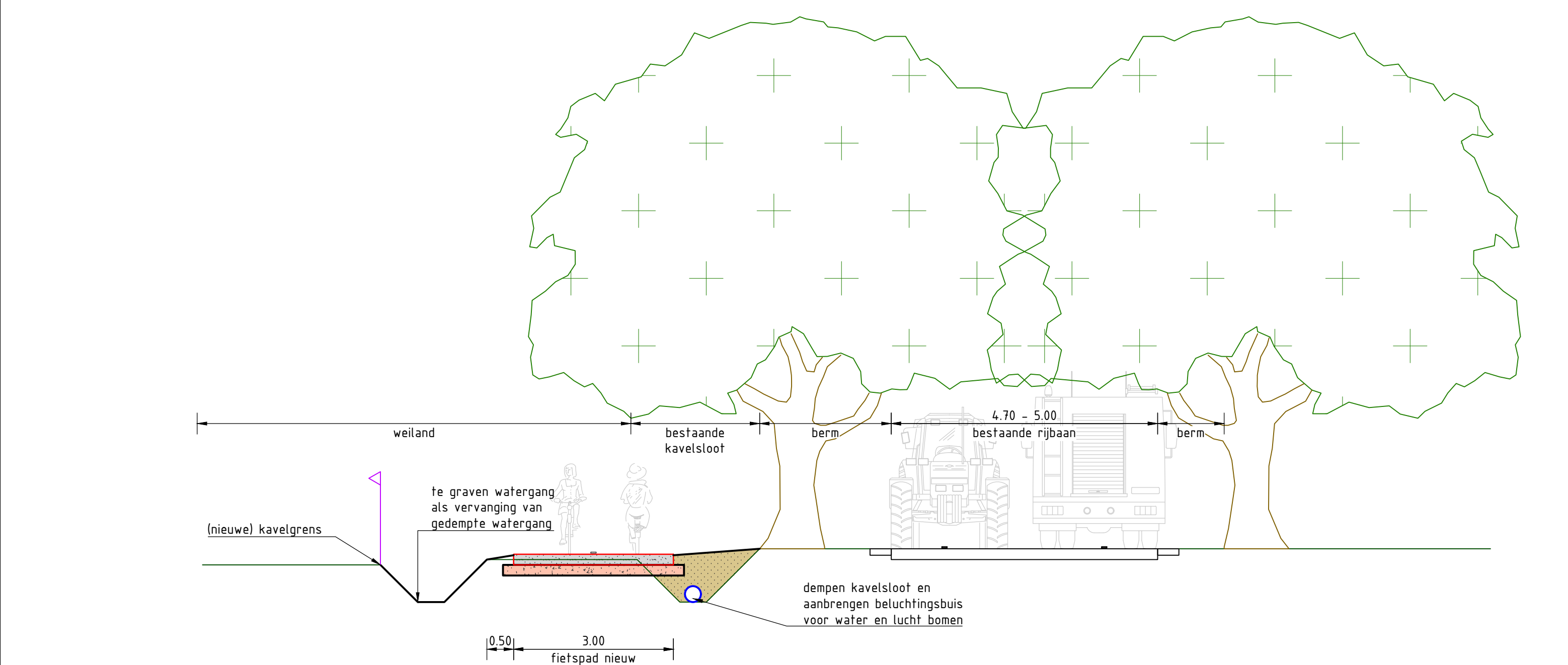
Principeprofiel B - Fietspad langs weiland of bebouwing
