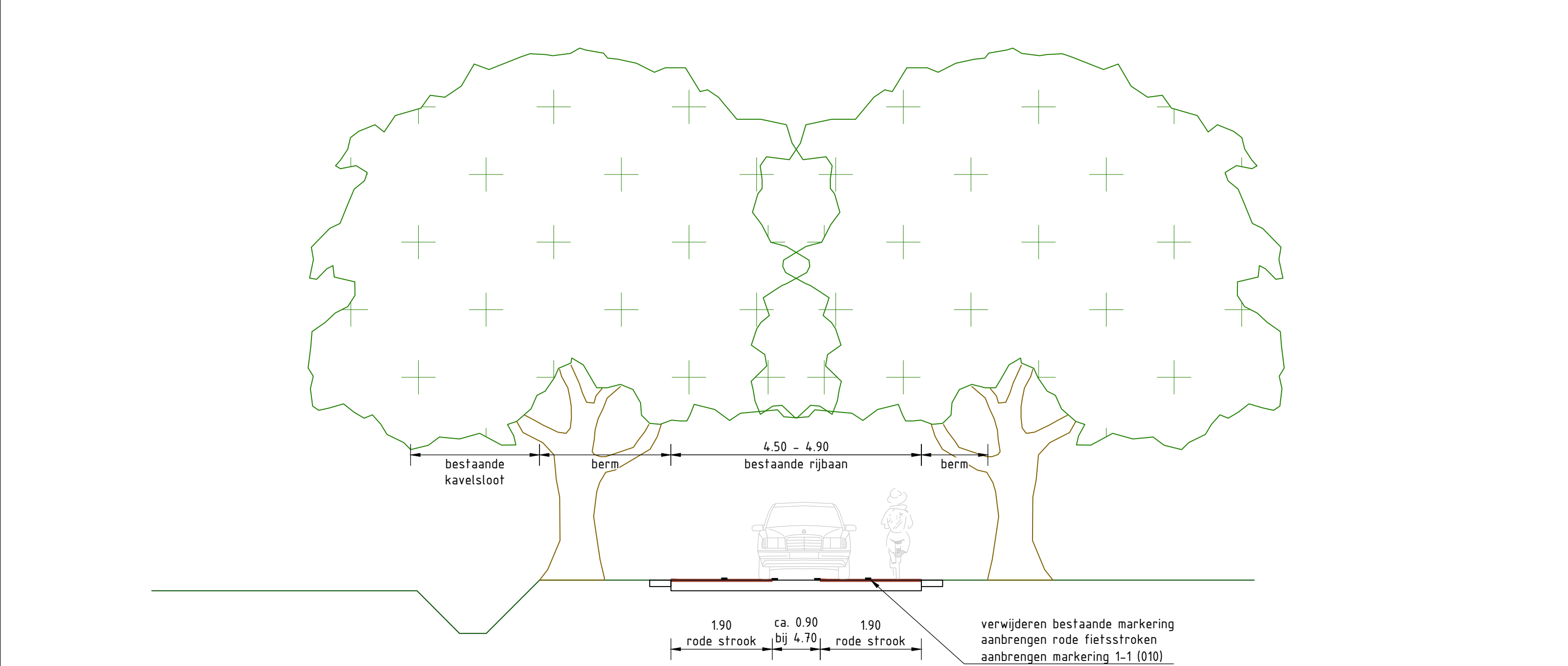
Principeprofiel E - Fietzers op de rijbaan
