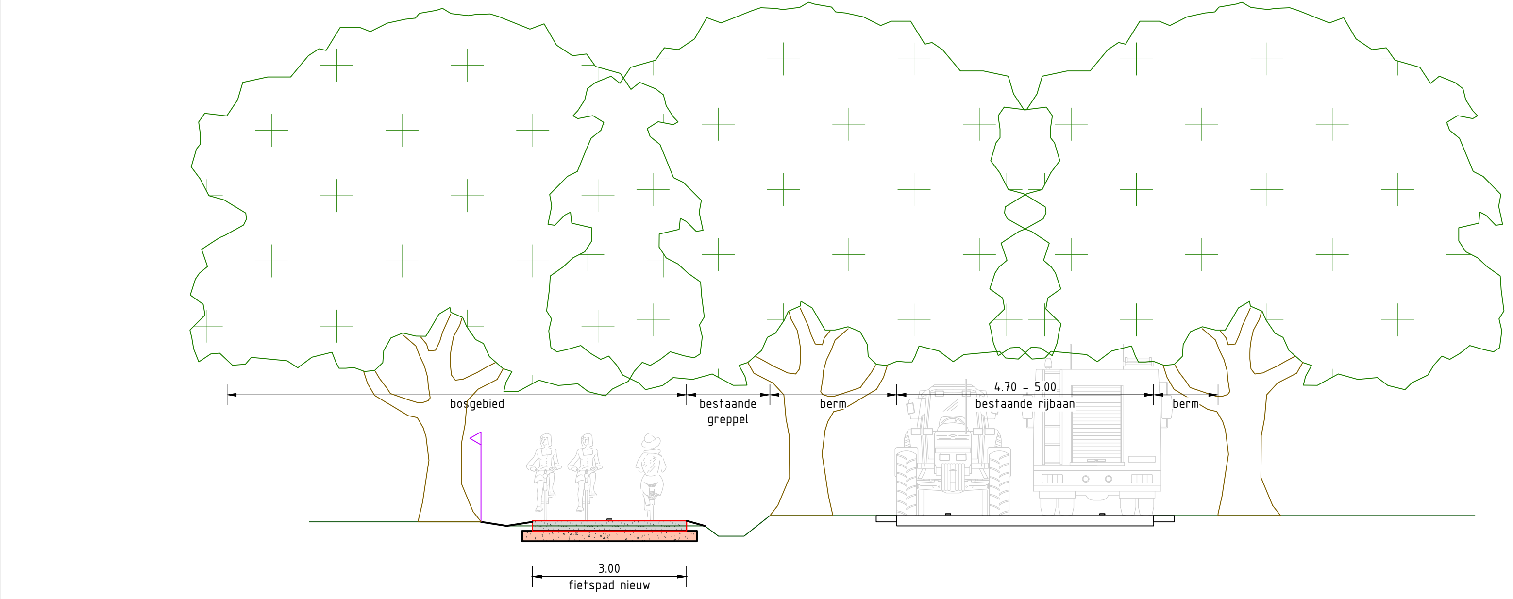
Principeprofiel C - Fietspad door bosgebied
