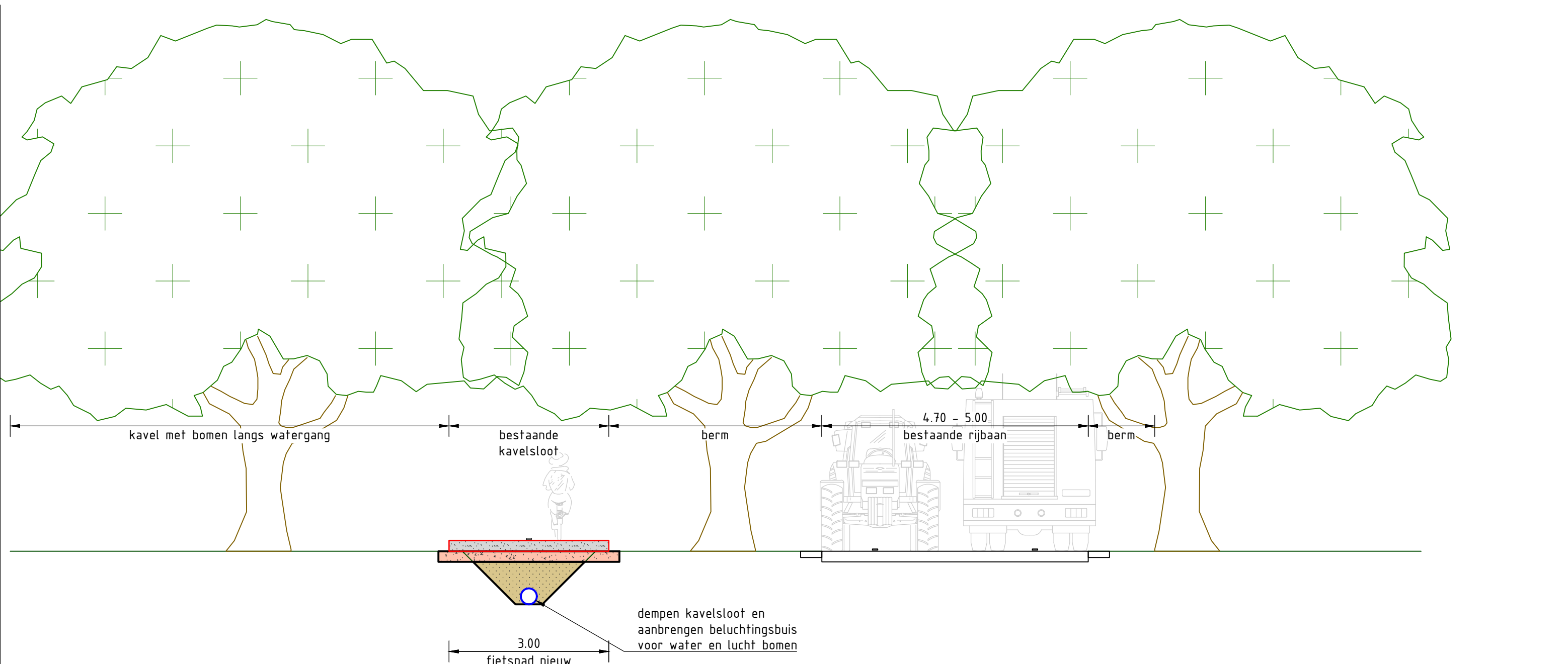
Principeprofiel A - Fietspad over bestaande kavelsloot
